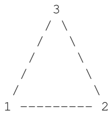
ESMF_MESHELEMENTTYPE_TRI
